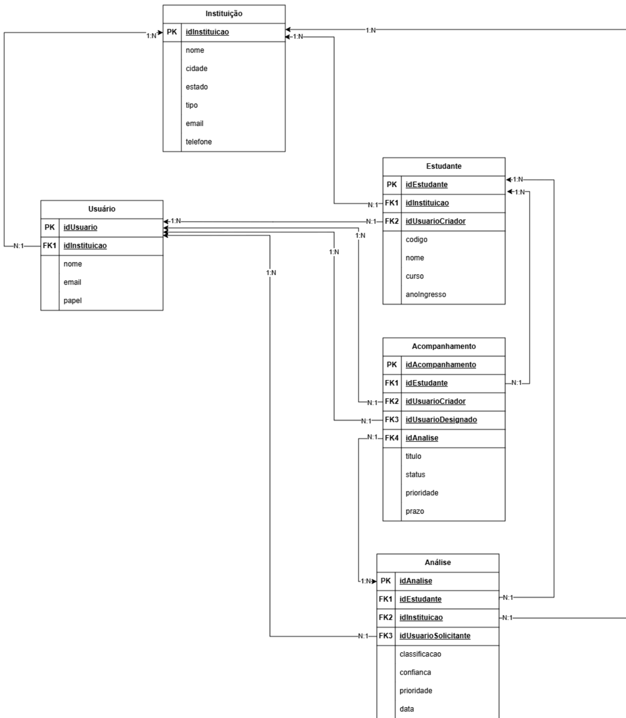
Imagem 4 - Diagrama lógico do Banco de dados do Backend-Project
