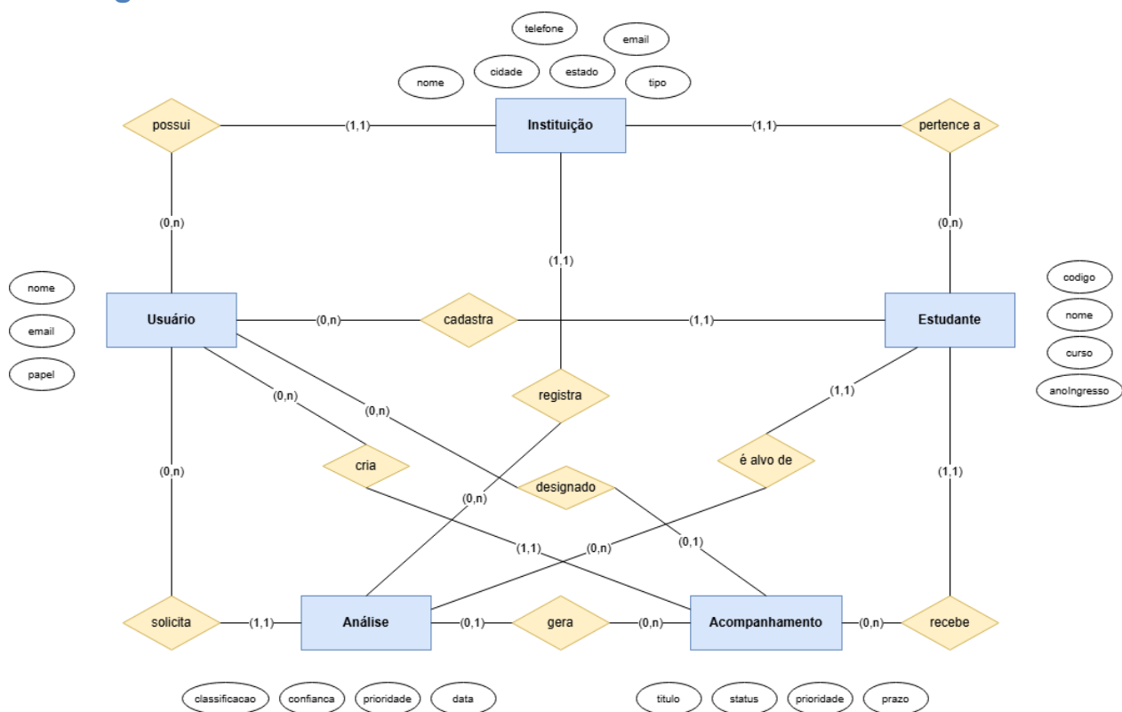
Imagem 3 - Diagrama conceitual do Banco de dados do Backend-Project
